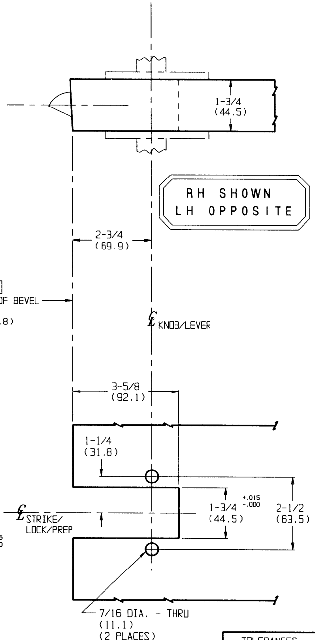
DOOR DETAIL
